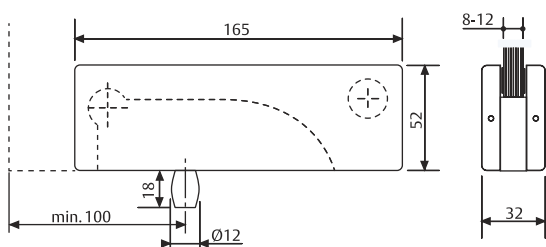
Dimensions
