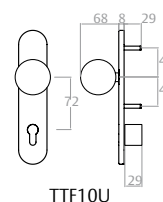
Pull knob
