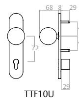
Pull knob
